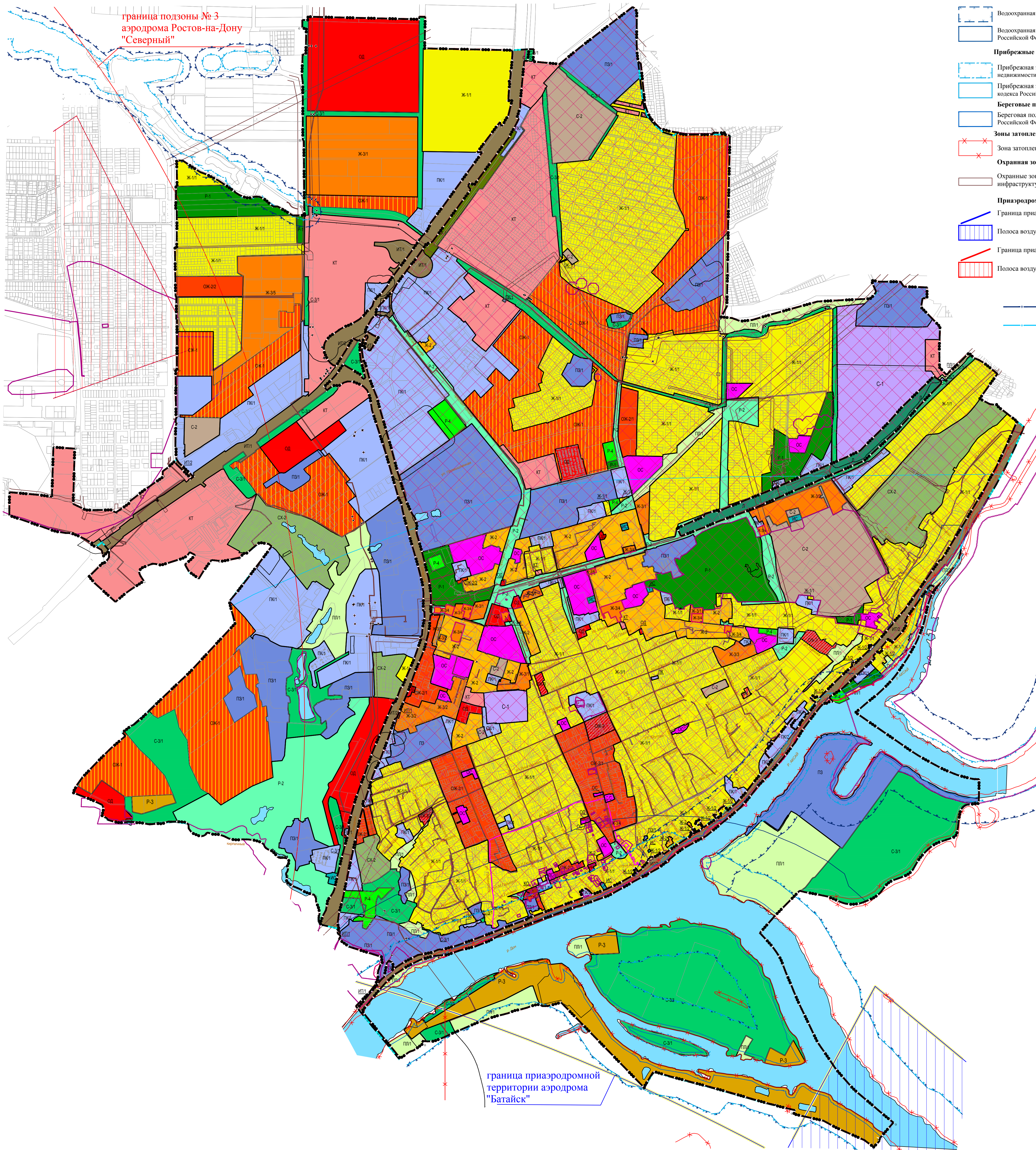
Профиль ограничения препятствий третьей подзоны аэродрома Ростов-на-Дону "Северный"
